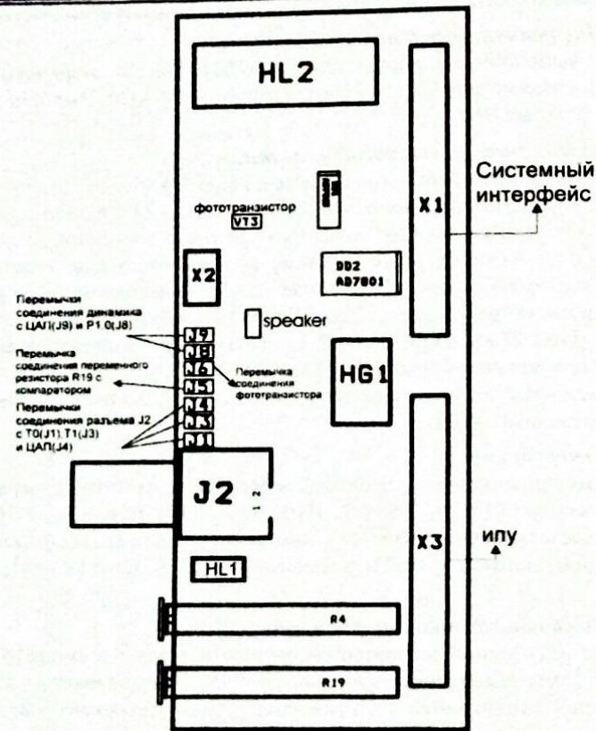
Рисунок 4. Схема расположения элементов платы расширения
