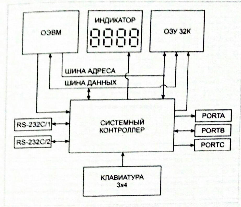
Рисунок 1. Структурная схема стенда
