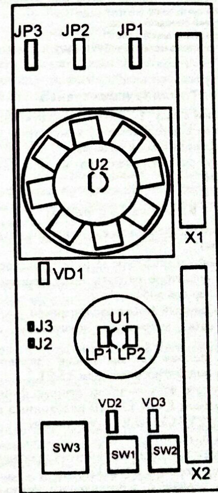
Рисунок 5. Схема расположения элементов платы расширения
